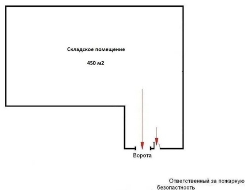
ПЛАН Эвакуации при пожаре (2-ой склад, 1-ый этаж)
