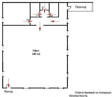
ПЛАН Эвакуации при пожаре (2-ой склад, 2-ой этаж)
